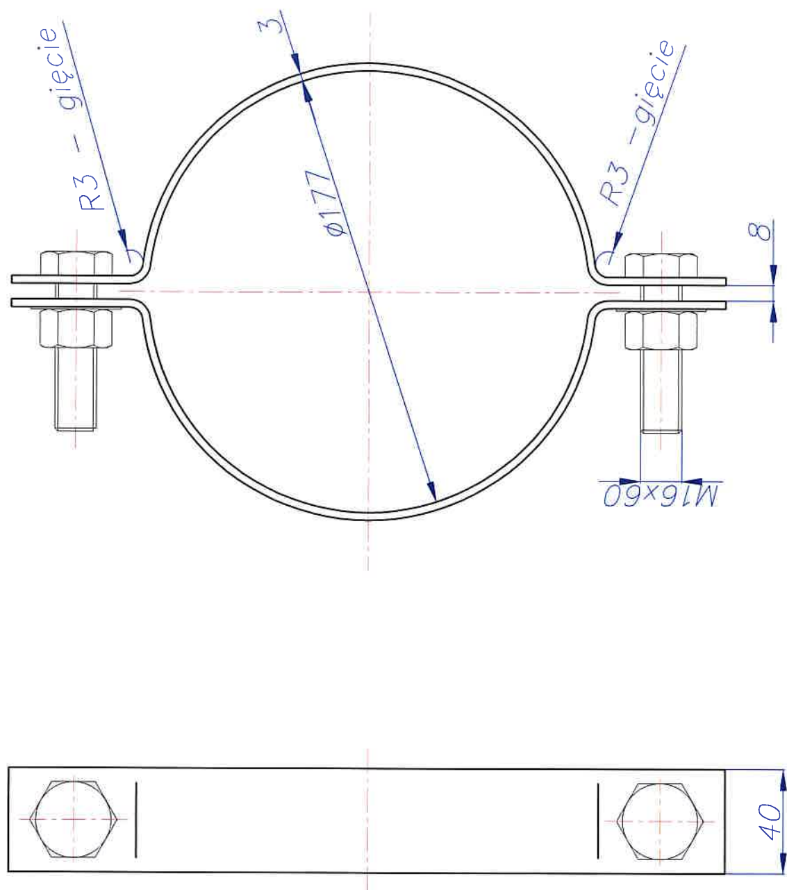
Obejma mocowania rur DN 150
